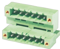
WJ2EDGRM-THT-5.0/5.08
