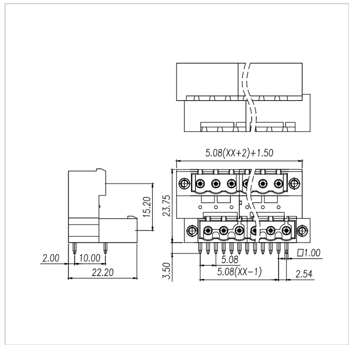
配件
