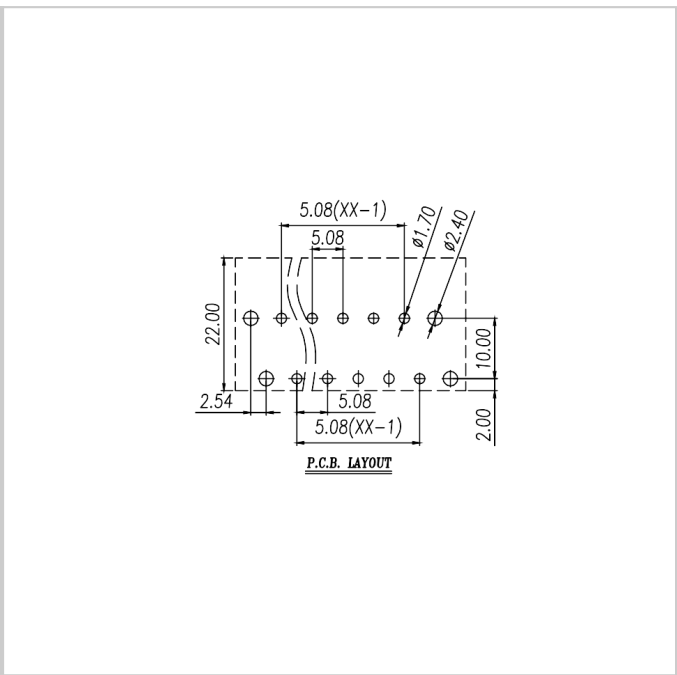
PCB开孔图
