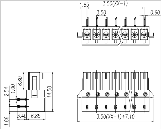
尺寸图
