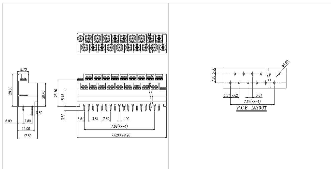
尺寸图
