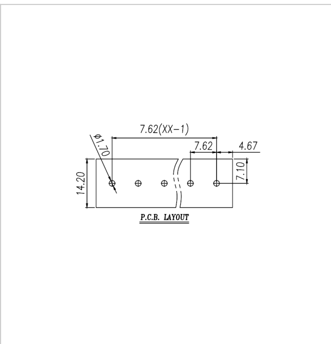
PCB开孔图
