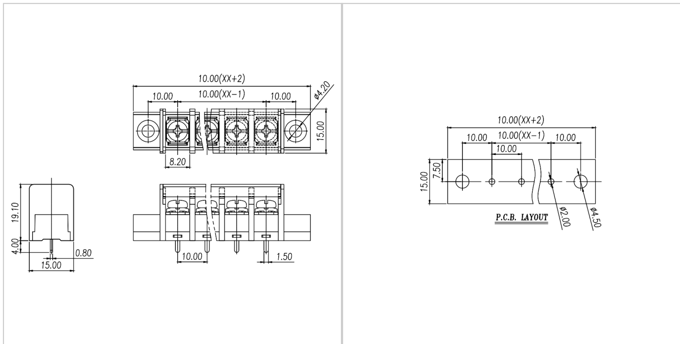
尺寸图
