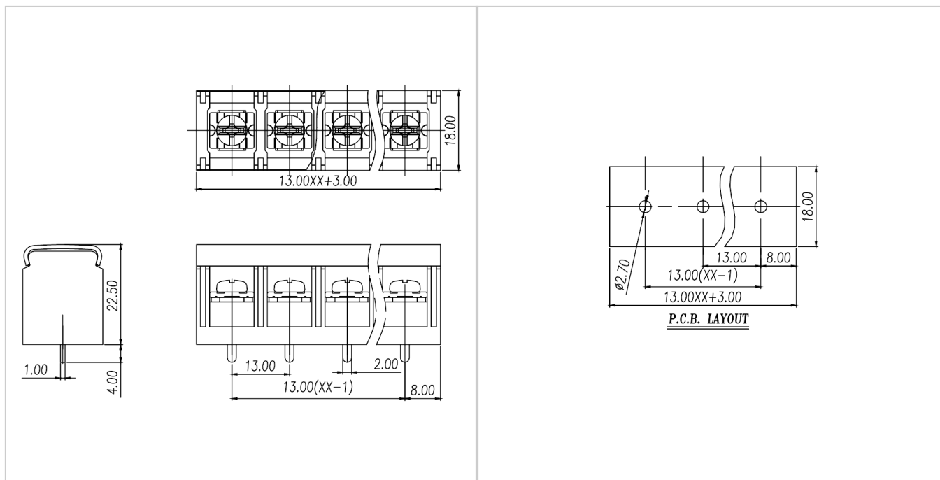
尺寸图
