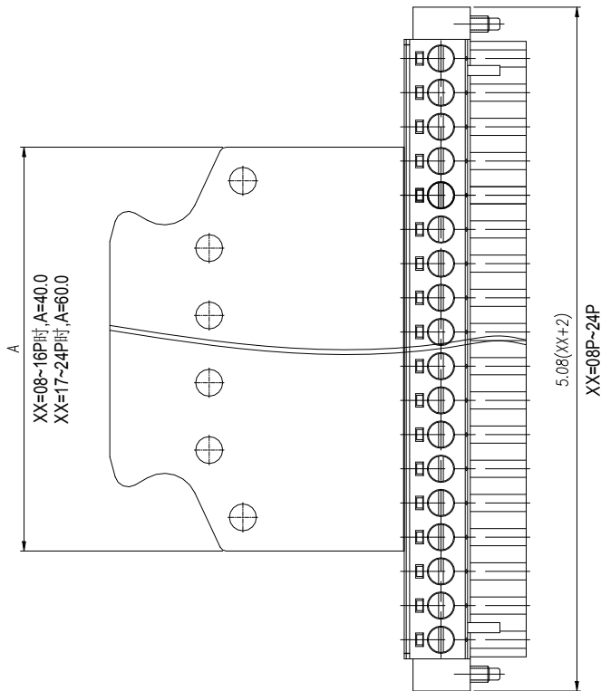
08~24P尺寸图
