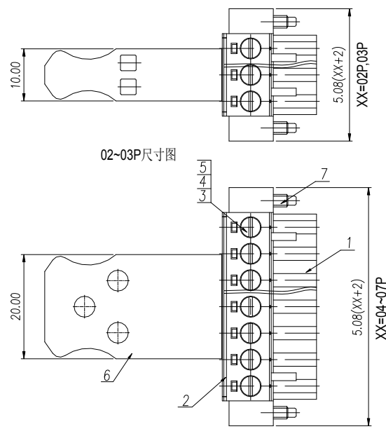
04~07P尺寸图
