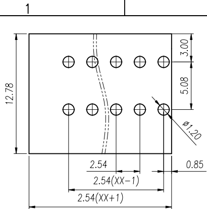
P.C.B. LAYOUT
