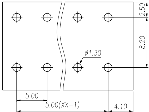
P.C.B. LAYOUT
