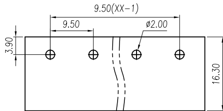
P.C.B. LAYOUT
