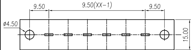
P.C.B. LAYOUT
